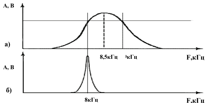
Рисунок 2 – АЧХ входного и выходного контуров (а) и АЧХ контура маркера (б)
