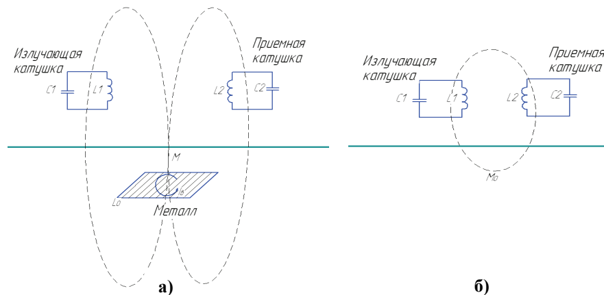
Рисунок 1 – Образование взаимной индуктивности при наличии металлического объекта (а) и при отсутствии (б)
