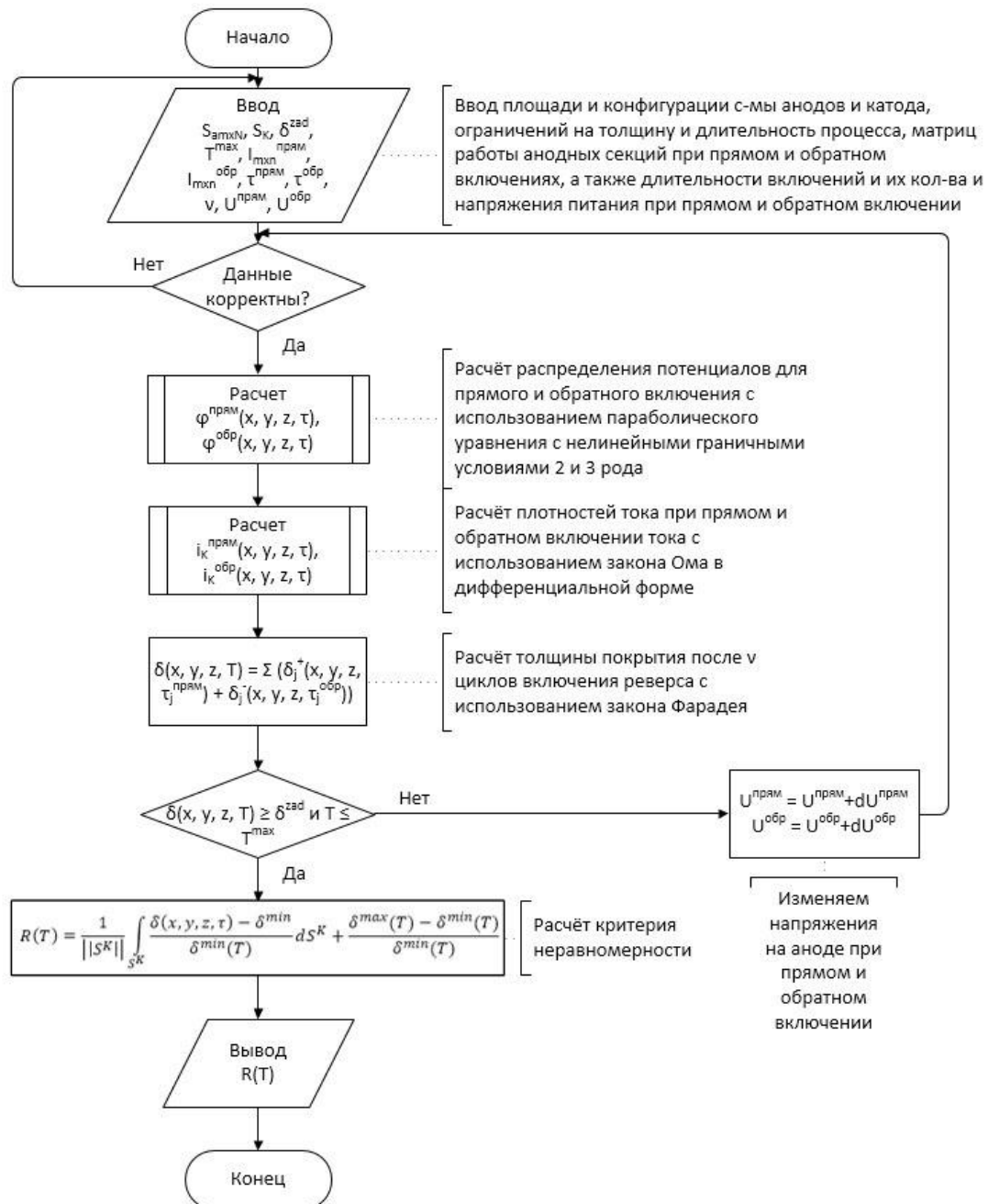
Рисунок 1 - Алгоритм расчета системы уравнений математической модели
