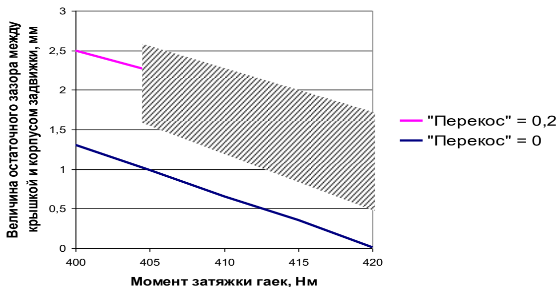
Рисунок 1 - Рациональная область соотношений величины зазора между корпусом и крышкой задвижки и моментом затяжки гаек
